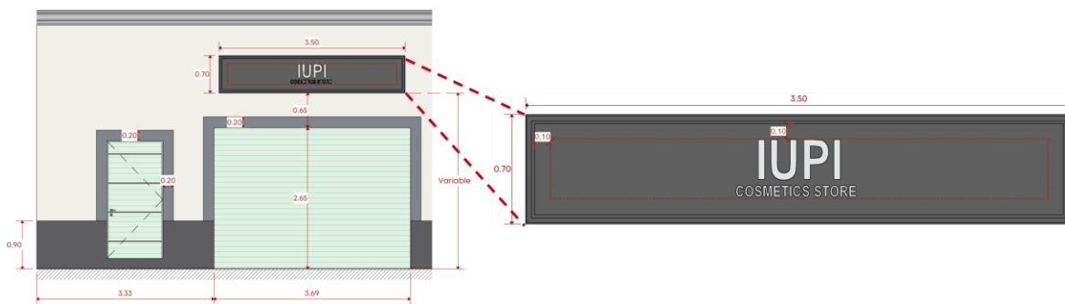
Figura 10. Letrero tipo 3
