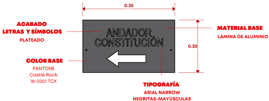
Figura 22. Detalle constructivo de señalización direccional
