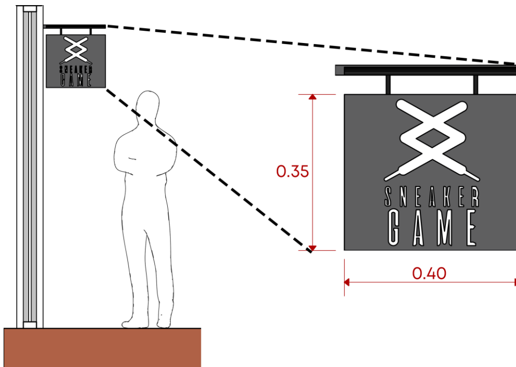
Figura 12. Letrero tipo 5
