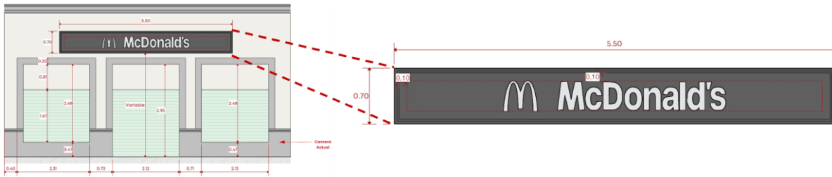
Figura 11. Letrero tipo 4
