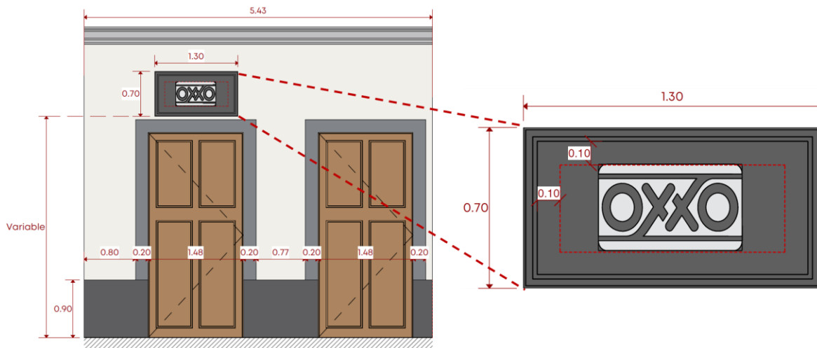
Figura 8. Letrero tipo 1
