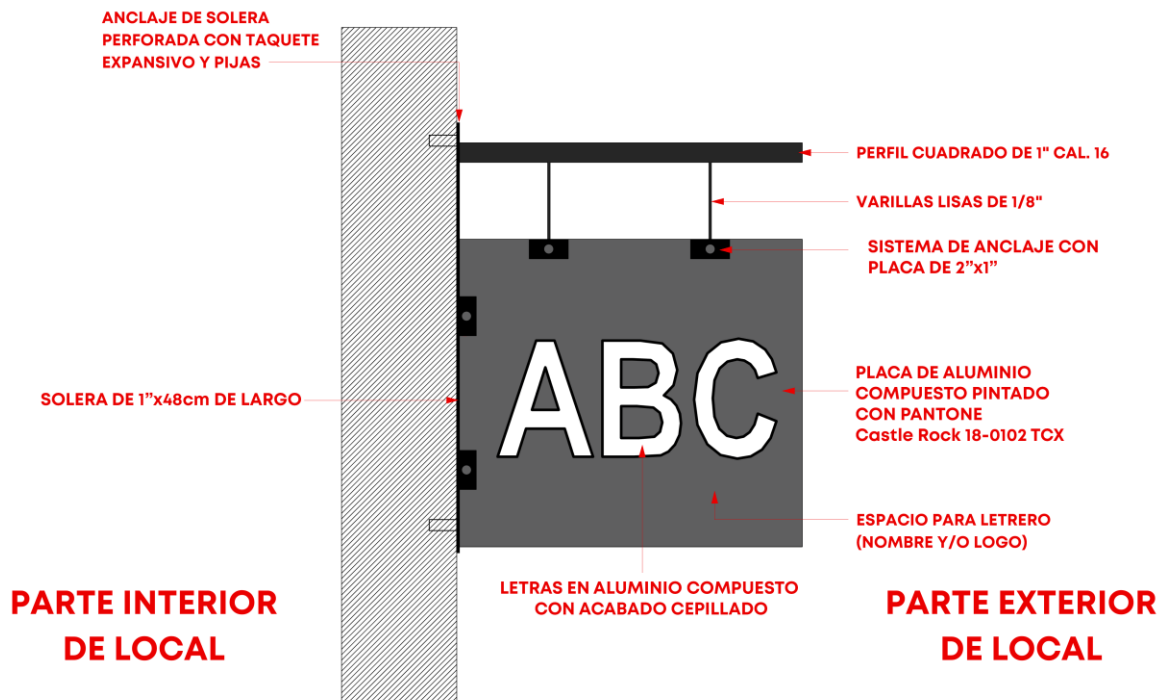
Figura 19. Detalle constructivo de anuncio denominativo tipo 5 anclado a muro
