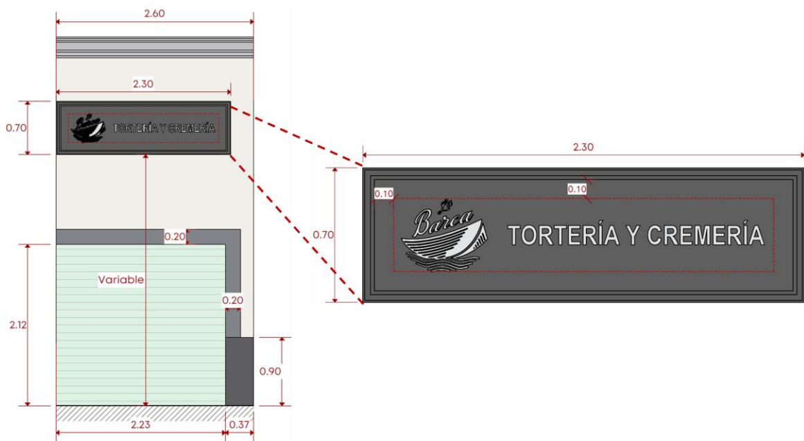
Figura 9. Letrero tipo 2
