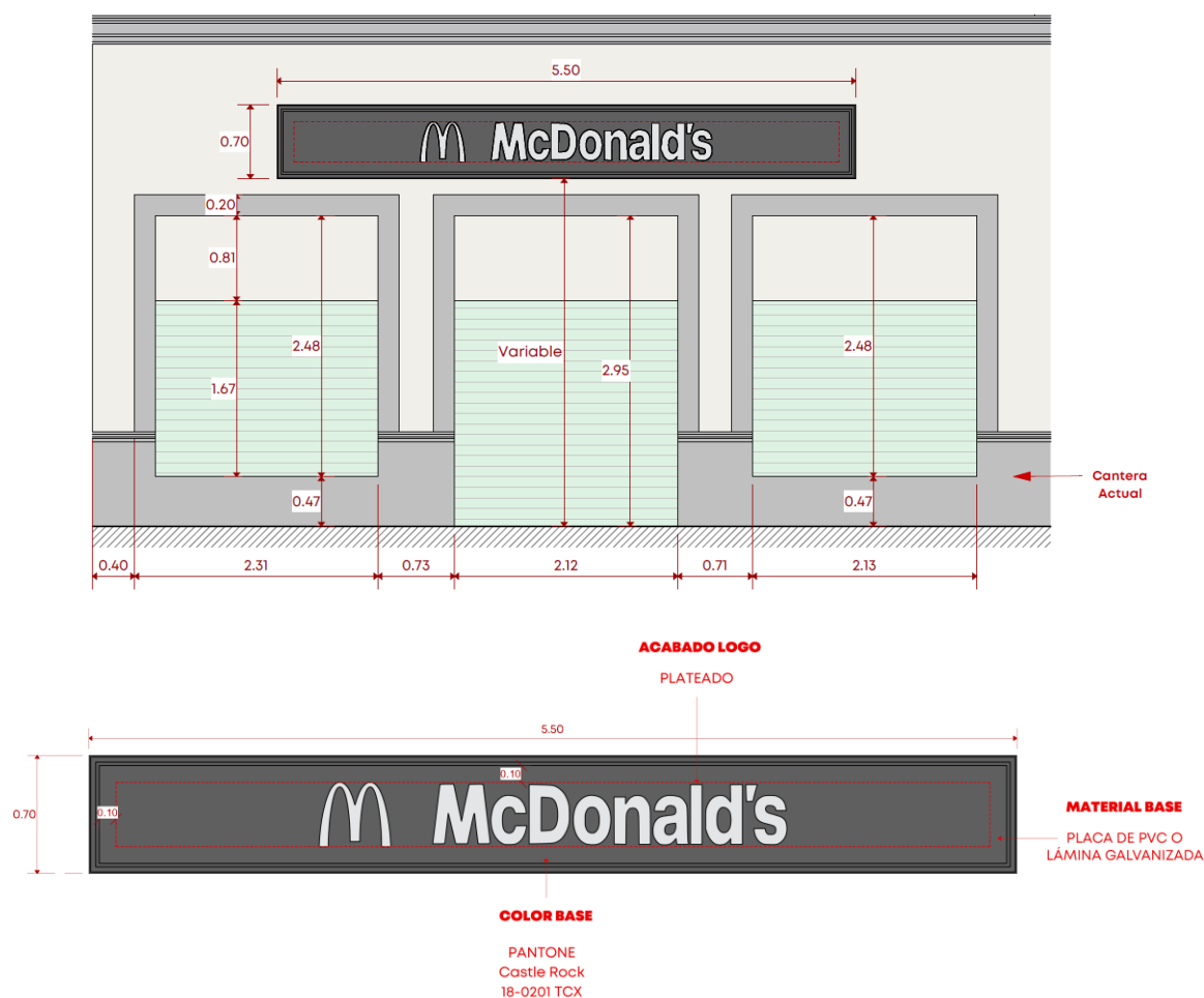
Figura 13. Letrero de marca registrada
