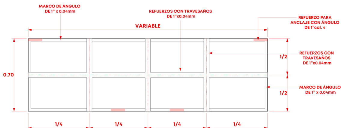
Figura 17. Detalle constructivo de bastidor anuncio denominativo tipo 1,2,3 y 4
